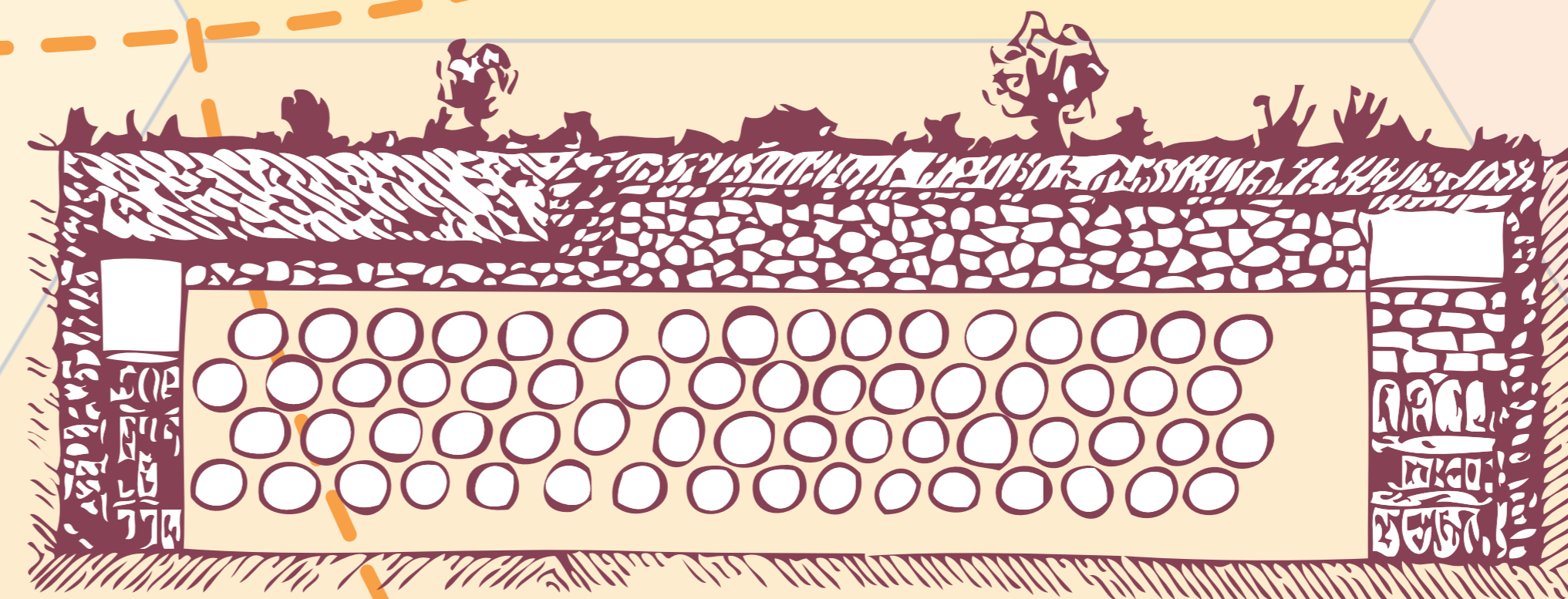
ALZADO-SECCIÓN LONGITUDINAL POSTERIOR. A-A
